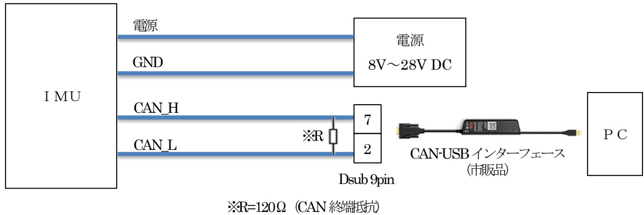
PC接続のブロック図
